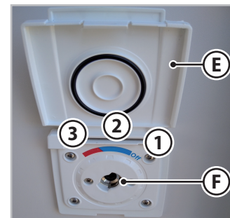
Fig. 6.40 - Prise de raccord de douche
