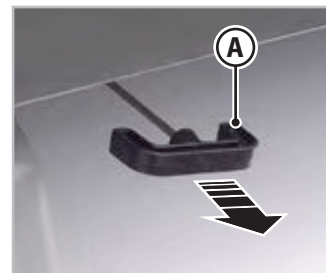
Fig.6.41 - Vanne de vidange des eaux grises
