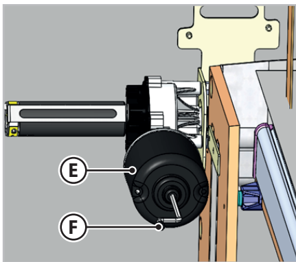
Fig.6.21 - Déblocage électrique du lit type B
