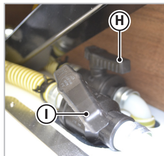
Fig. 6.39 - Vanne de vidange d'eau propre double plancher
