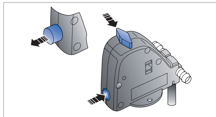
Fig. 6.47 - Soupape de sécurité Combi
